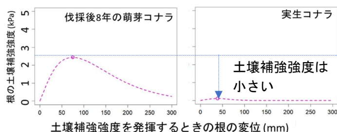
図3 萌芽コナラと実生コナラの根の土壌補強強度の違い
