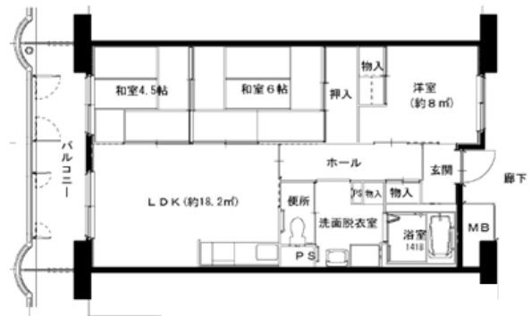
間取り図
