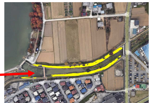
両岸に遮光シートを設置（黄色部分）
