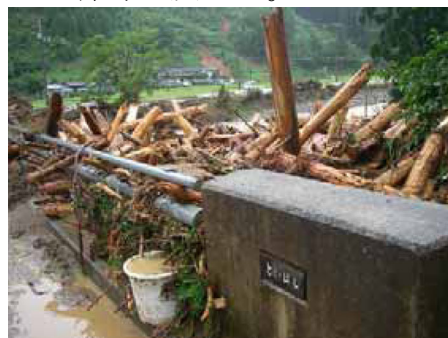
流木による橋梁箇所での閉塞状況
