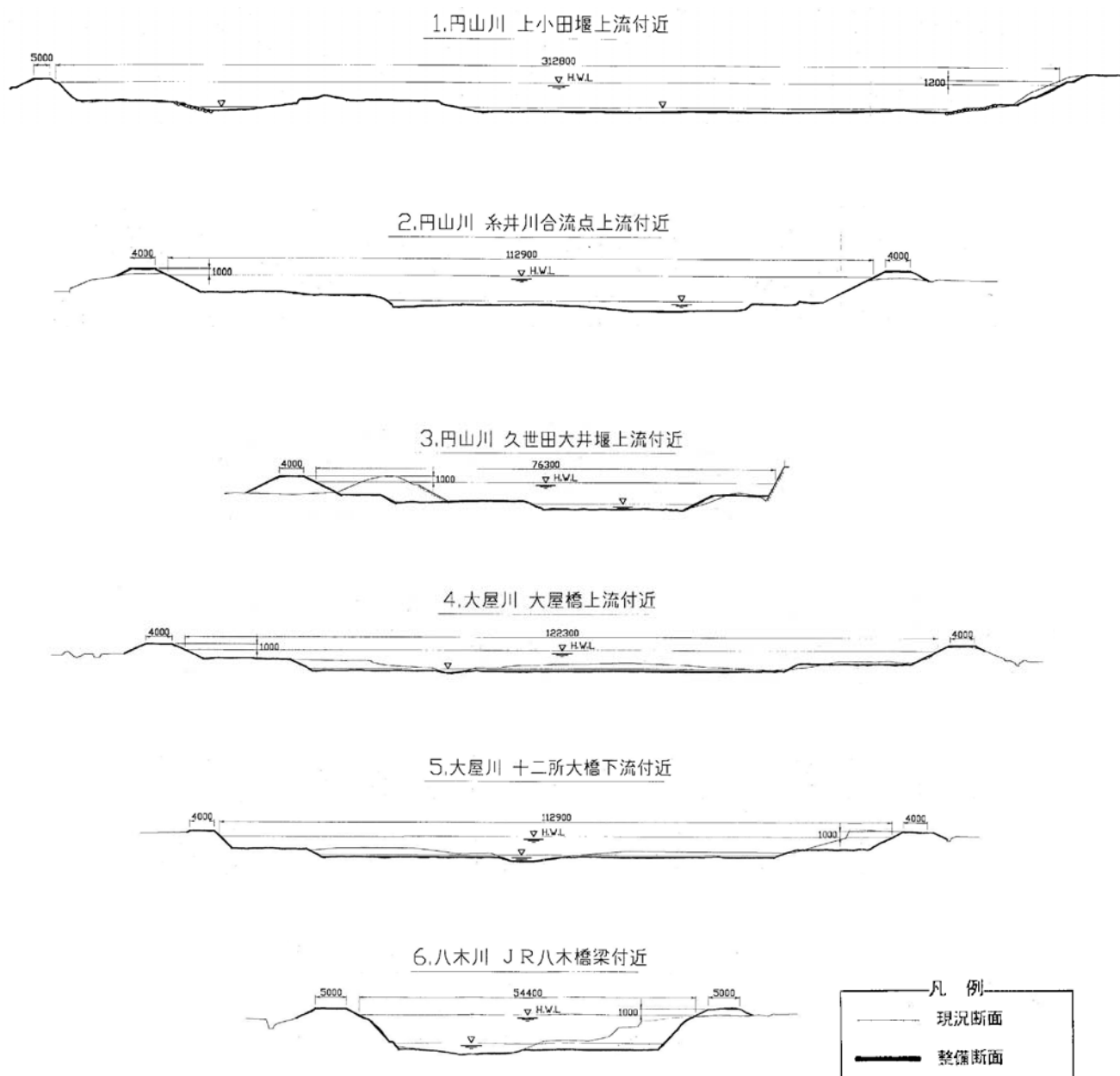
図 1.3.6 円山川上流圏域（県管理区間）河川整備計画における標準断面の例
