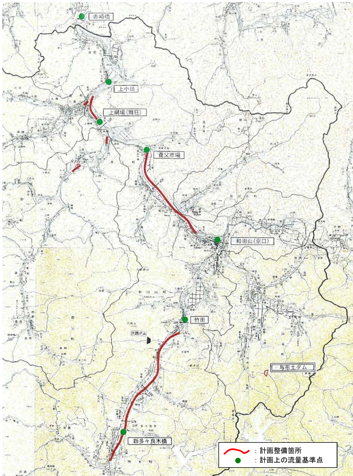
図 1.3.7 円山川上流圏域（県管理区間）河川整備計画における整備箇所位置図
