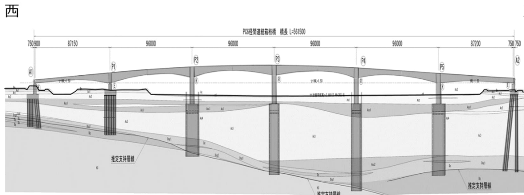
断面図
