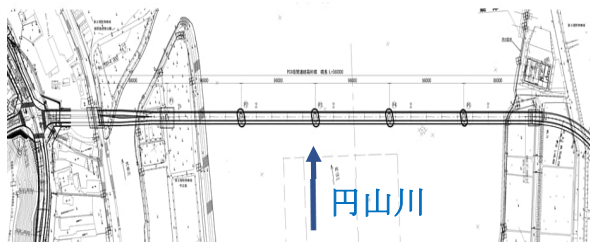
平面図
