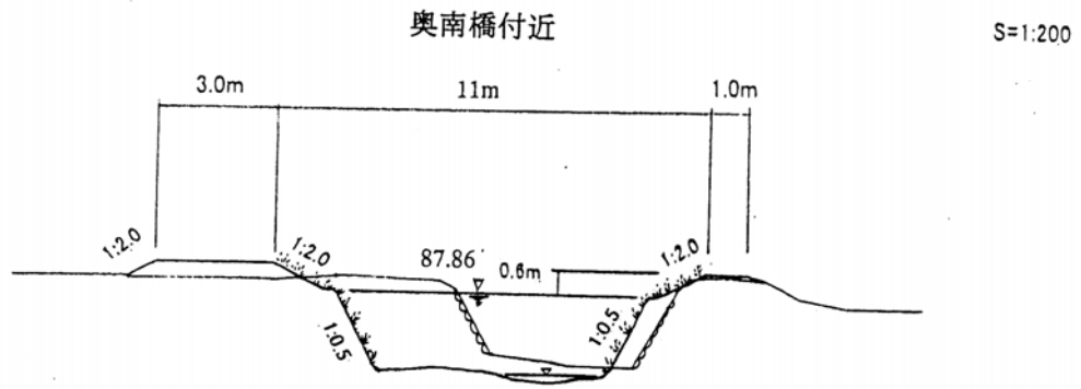
岩屋谷川代表横断面図
