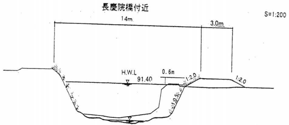
石戸川代表横断面図
