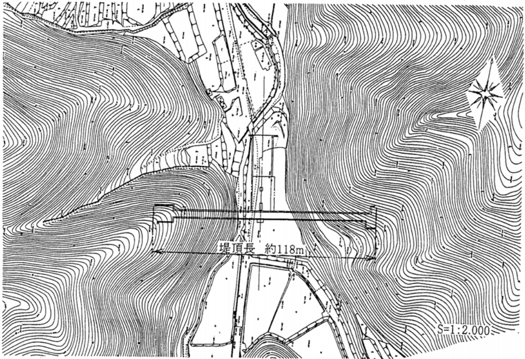
平面図
