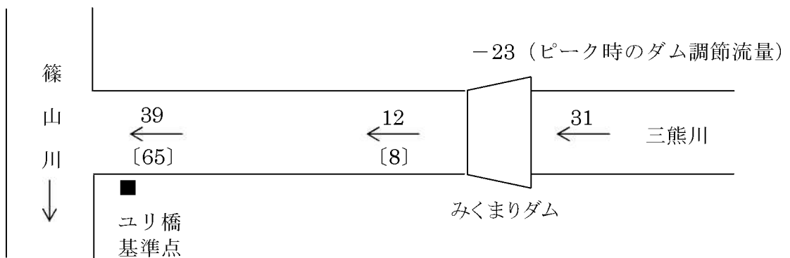
図 2.1.8 計画高水流量配分図
