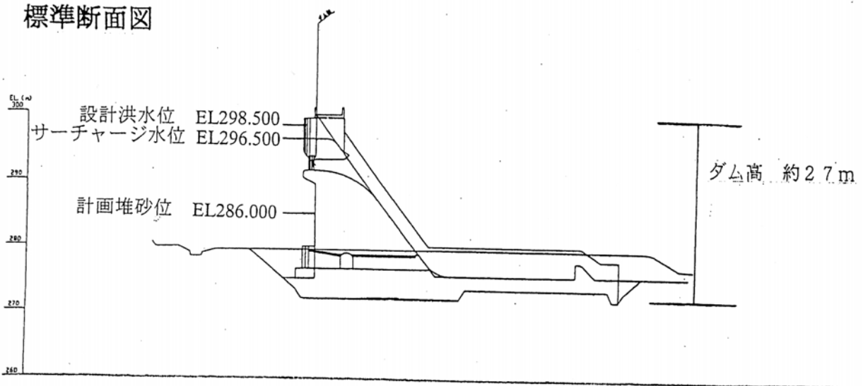
図-2.17 みくまりダム
