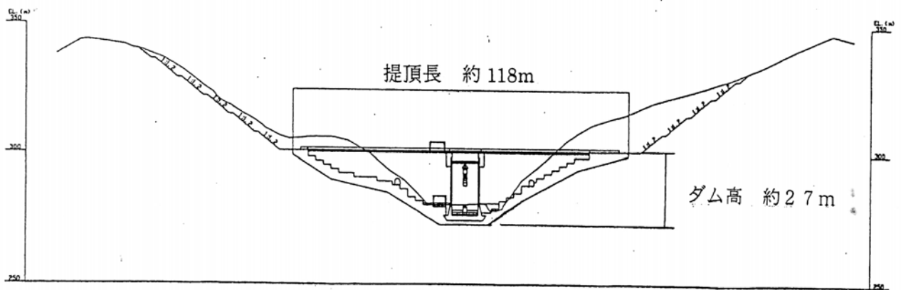
下流面図
