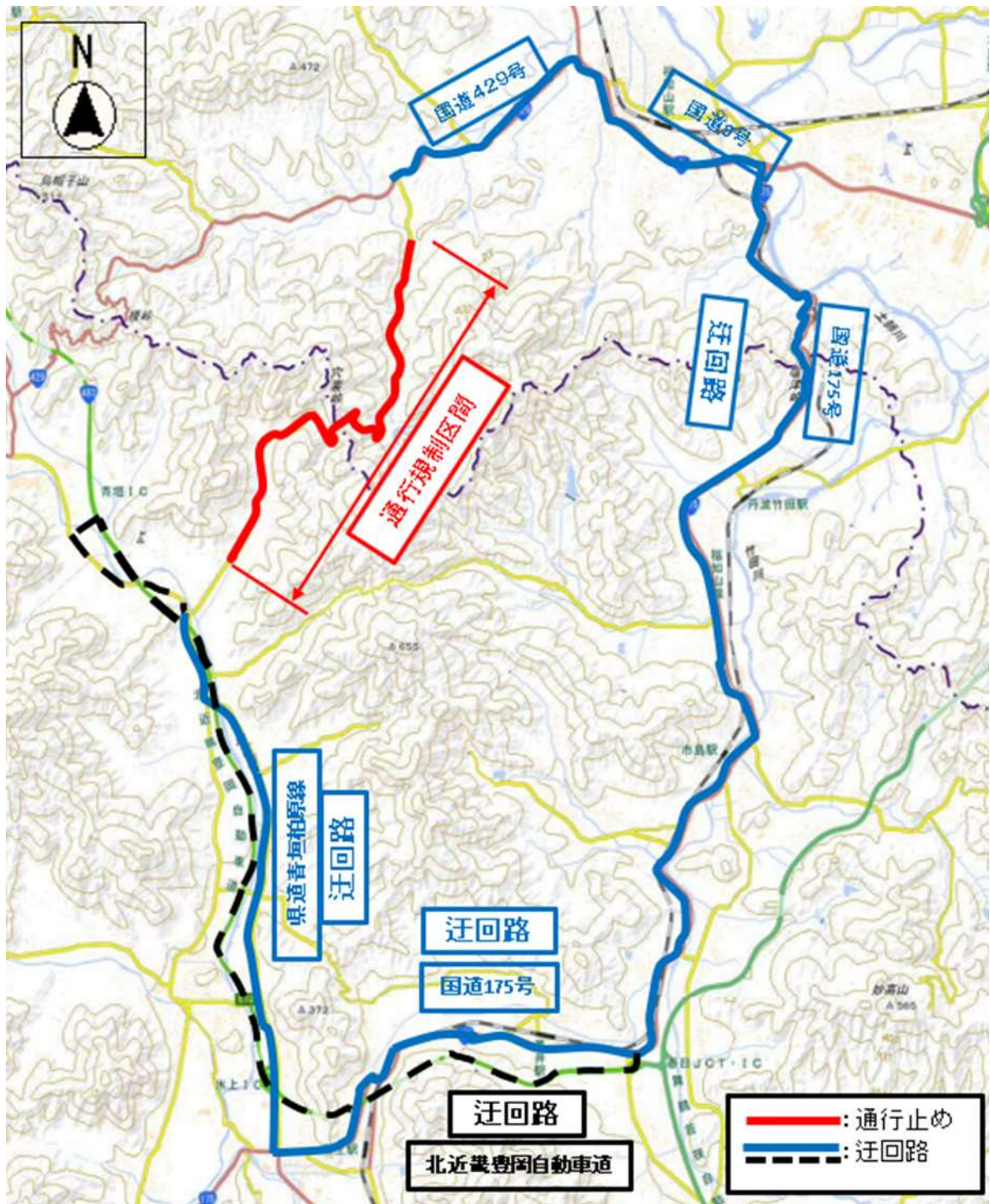
迂回路図
