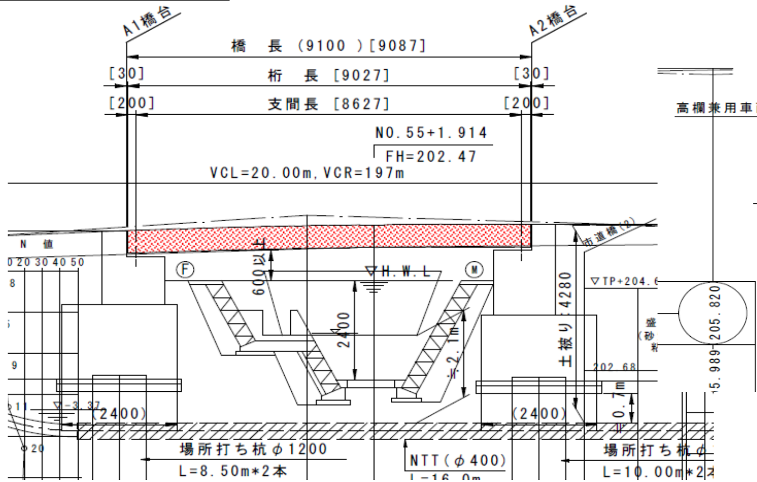
上部工構造一般図
