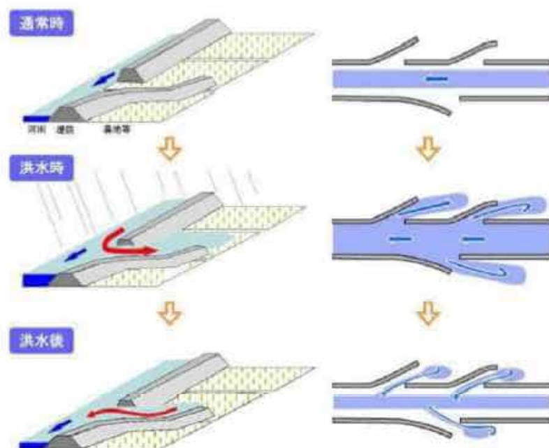
図 5-4 霞堤のイメージ
