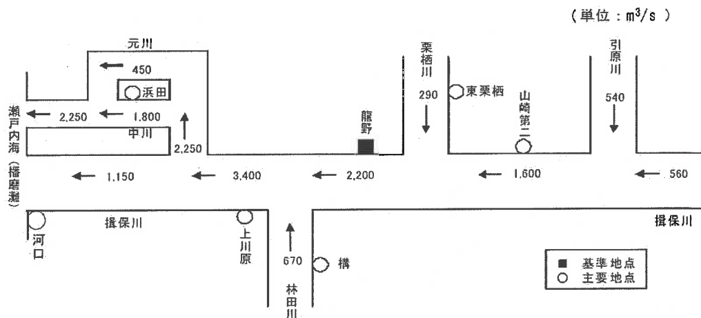
図 4-1 流量配分図(整備計画目標流量)
