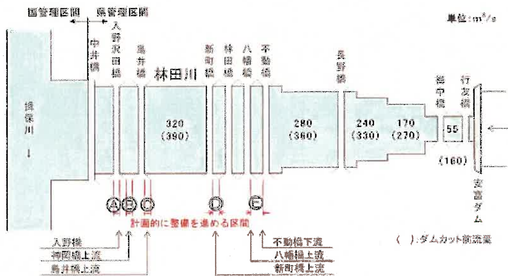
図 4-27 目標流量流量配分図 (林田川)
