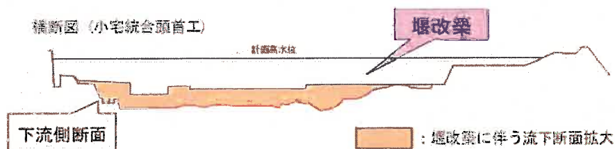
図 4-6 河川整備イメージ（髯崎地区）
