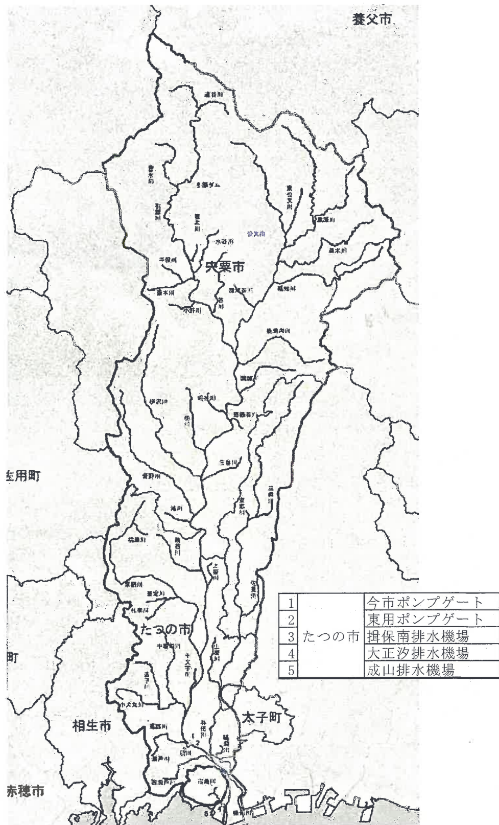
図 5-14 ポンプ位置図
