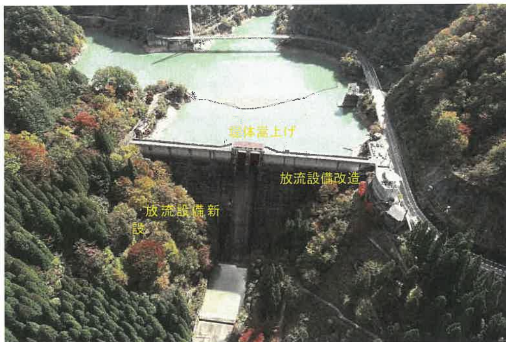
図 0-34 ダム再生後イメージ
