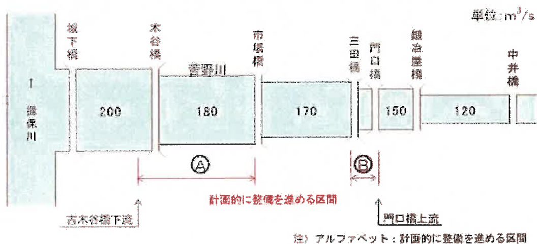
図 4-31 目標流量流量配分図 (菅野川)
