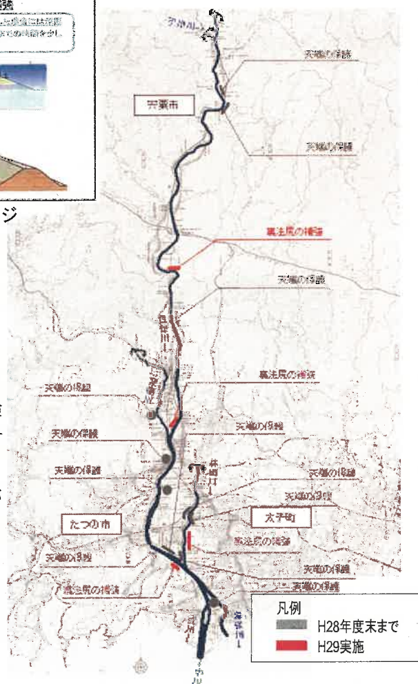
図 4-34 危機管理型ハード対策位置図
