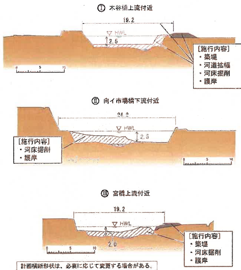
図 4-32 整備横断イメージ図 (菅野川)
