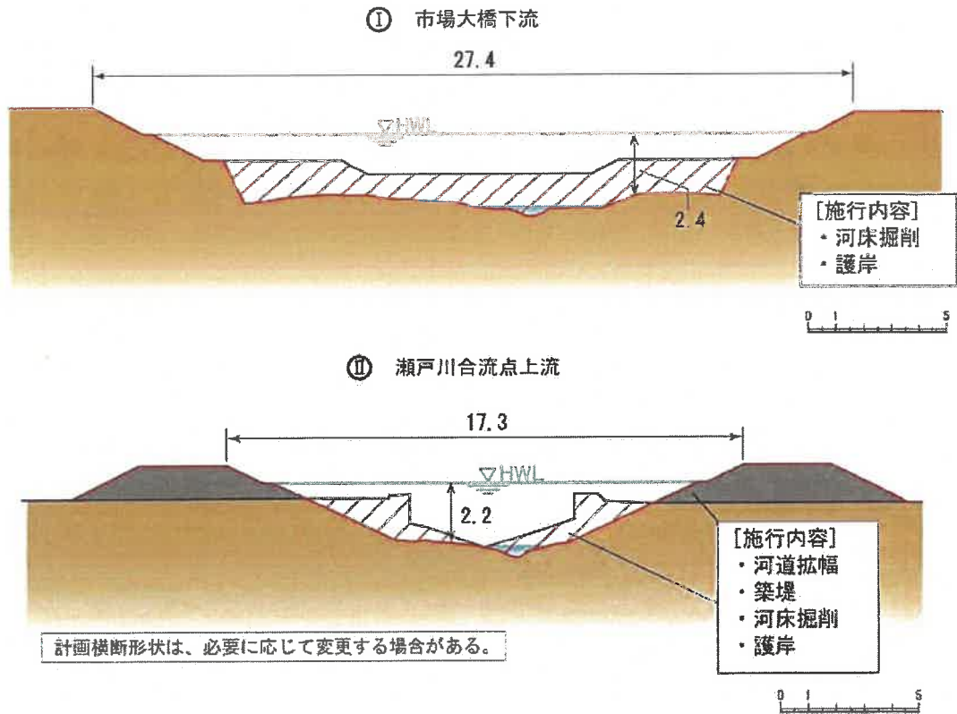
図 4-26 整備横断イメージ図 (前川)
