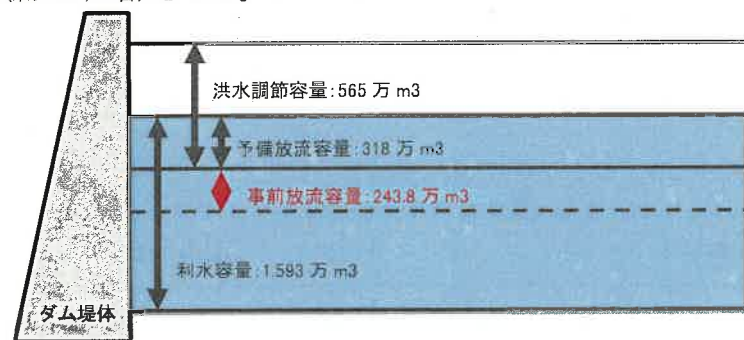
図 5-13 引原ダムの事前放流容量
