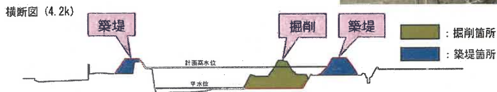
図 4-21 河川整備イメージ (段之上地区)
