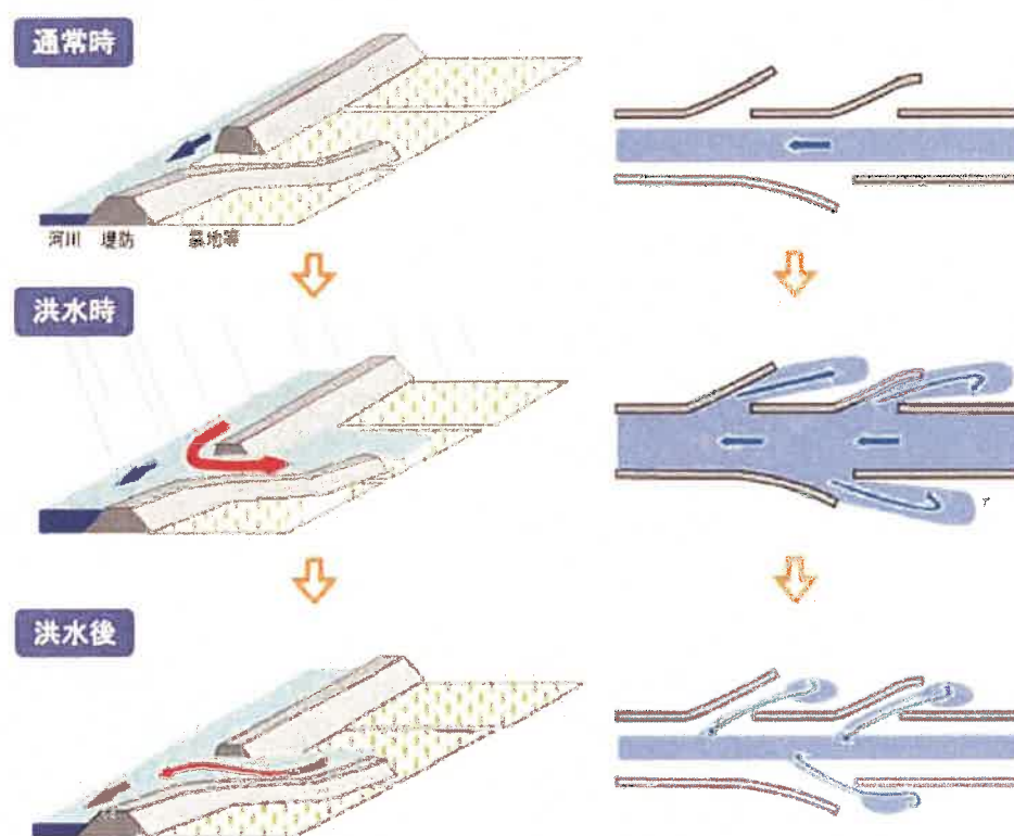
図 5-15 霞堤のイメージ
