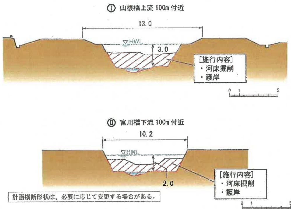
図 4-30 整備横断イメージ図 (山根川)
