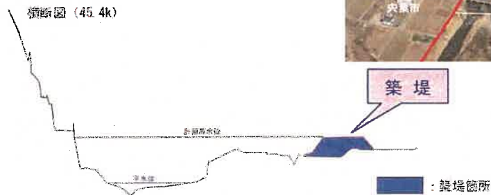
図 4-17 河川整備イメージ (中安積地区)
