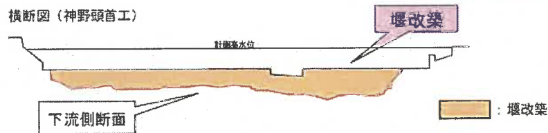
図 4-14 河川整備イメージ (安黒地区)
