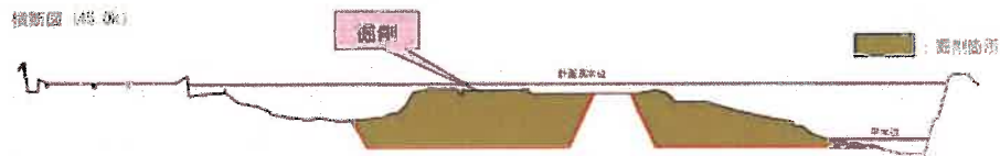
図 4-16 河川整備イメージ (曲里地区)
