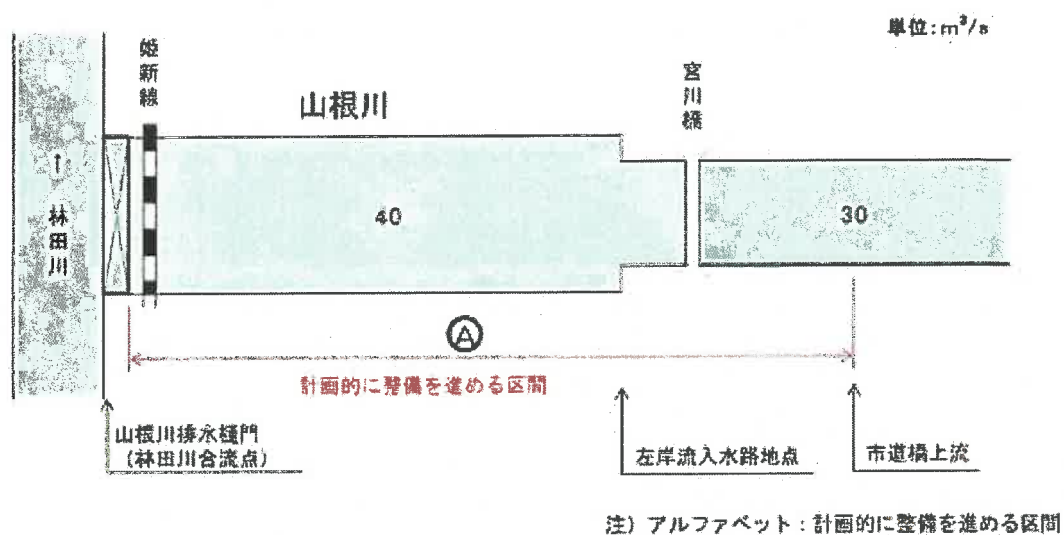
図 4-29 目標流量流量配分図 (山根川)
