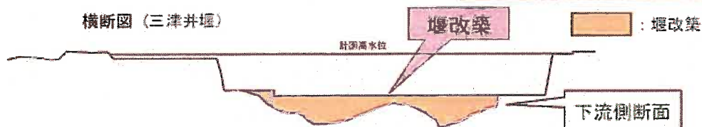
図 4-12 河川整備イメージ (岸田地区)
