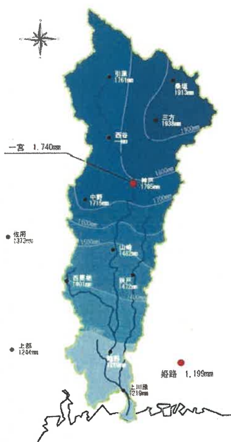
図1-7 年平均等雨量線図 (S56～H22年の30年平均)
