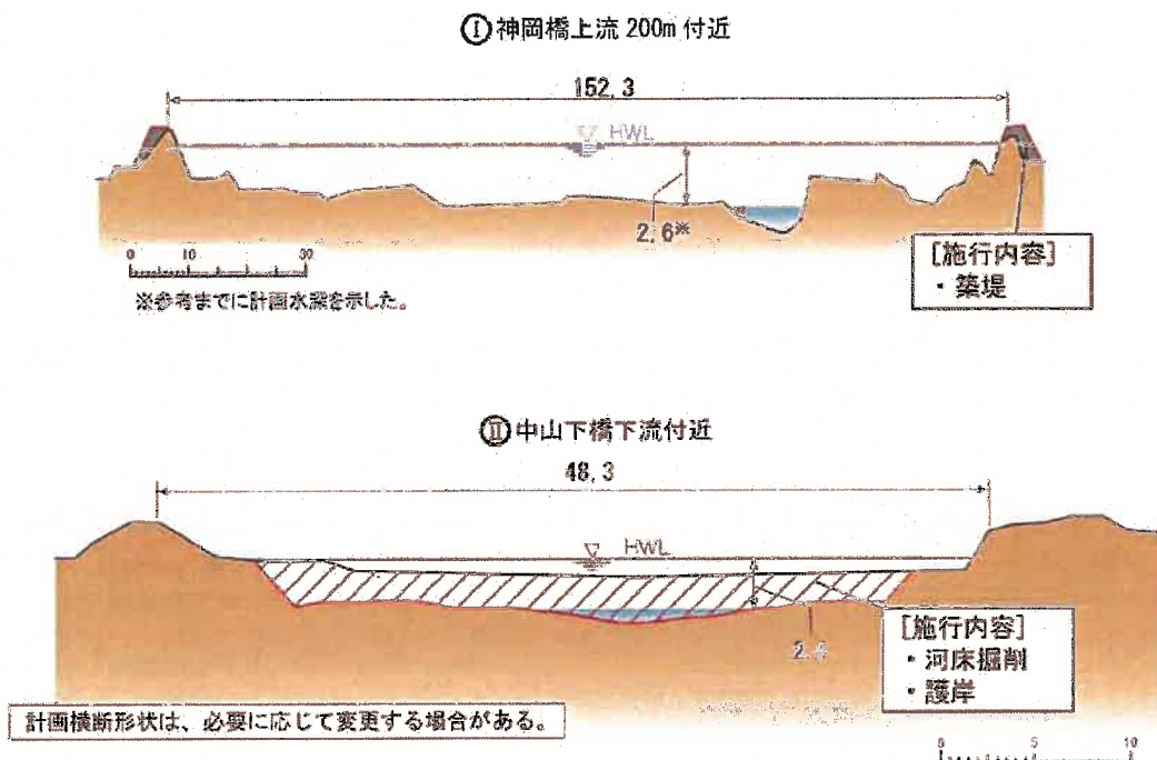
図 4-28 整備横断イメージ図 (林田川)
